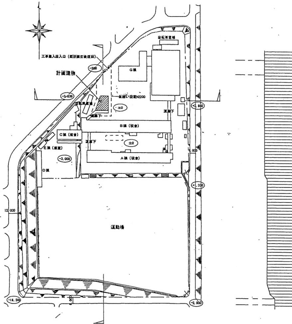
配置図 1/1500
